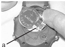
Рис. 113 - ИЗВЛЕЧЕНИЕ БАТАРЕЙКИ
