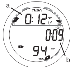
Рис. 26 – ВРЕМЯ (ПОГРУЖЕНИЕ)
