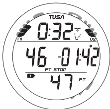
Рис. 68 - DS ОСНОВНОЙ
